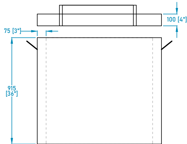
ELEVATION - 3' & LID
